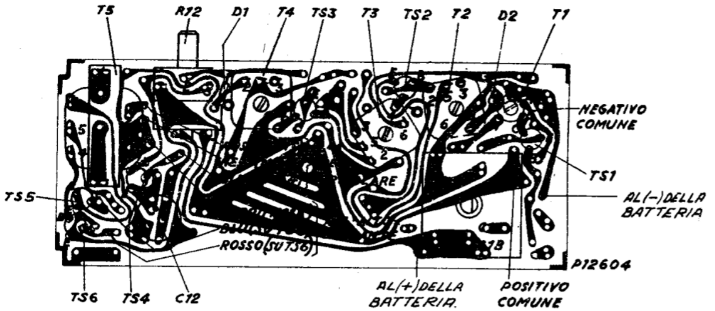
Piastra del circuito stampato: i componenti elettrici sono visti per trasparenza
